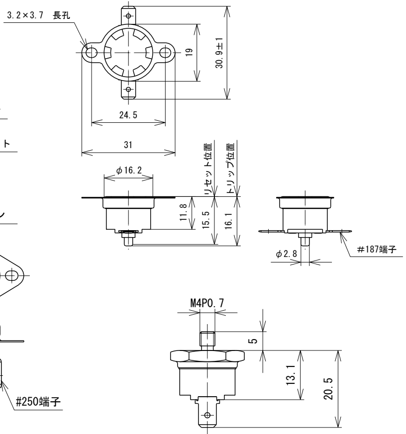
05 寸法図
